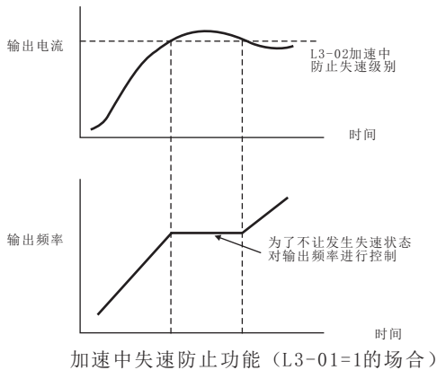
加速中失速防止功能 (L3-01=1的场合)
